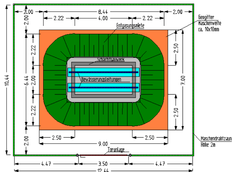
Grundriß Entgasungsfenster
